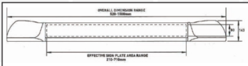
A6654.000 type 1250mm 4 module
